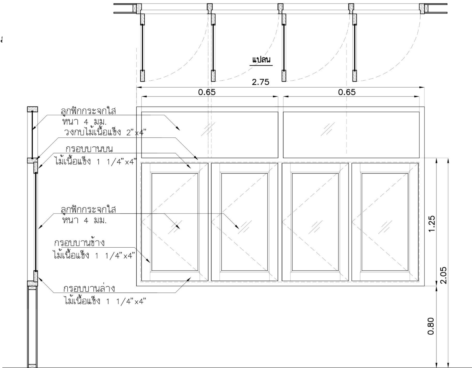
รูปตัด หน้าต่างบานไม้เปิดชุดต่อเนื่อง ชนิดบานลูกฟักกระจกช่องแสงบน
