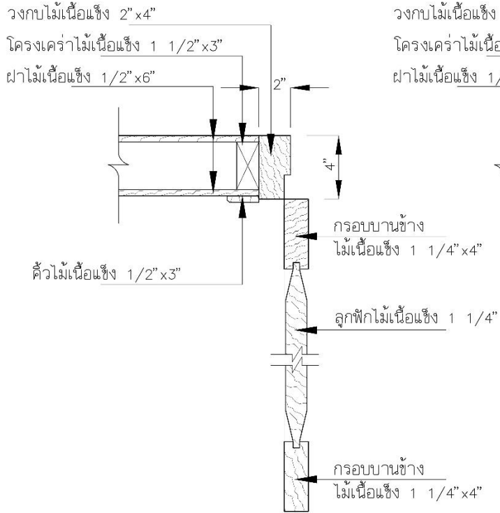
แบบขยายประตู ประตูบานลูกฟิกไม้
