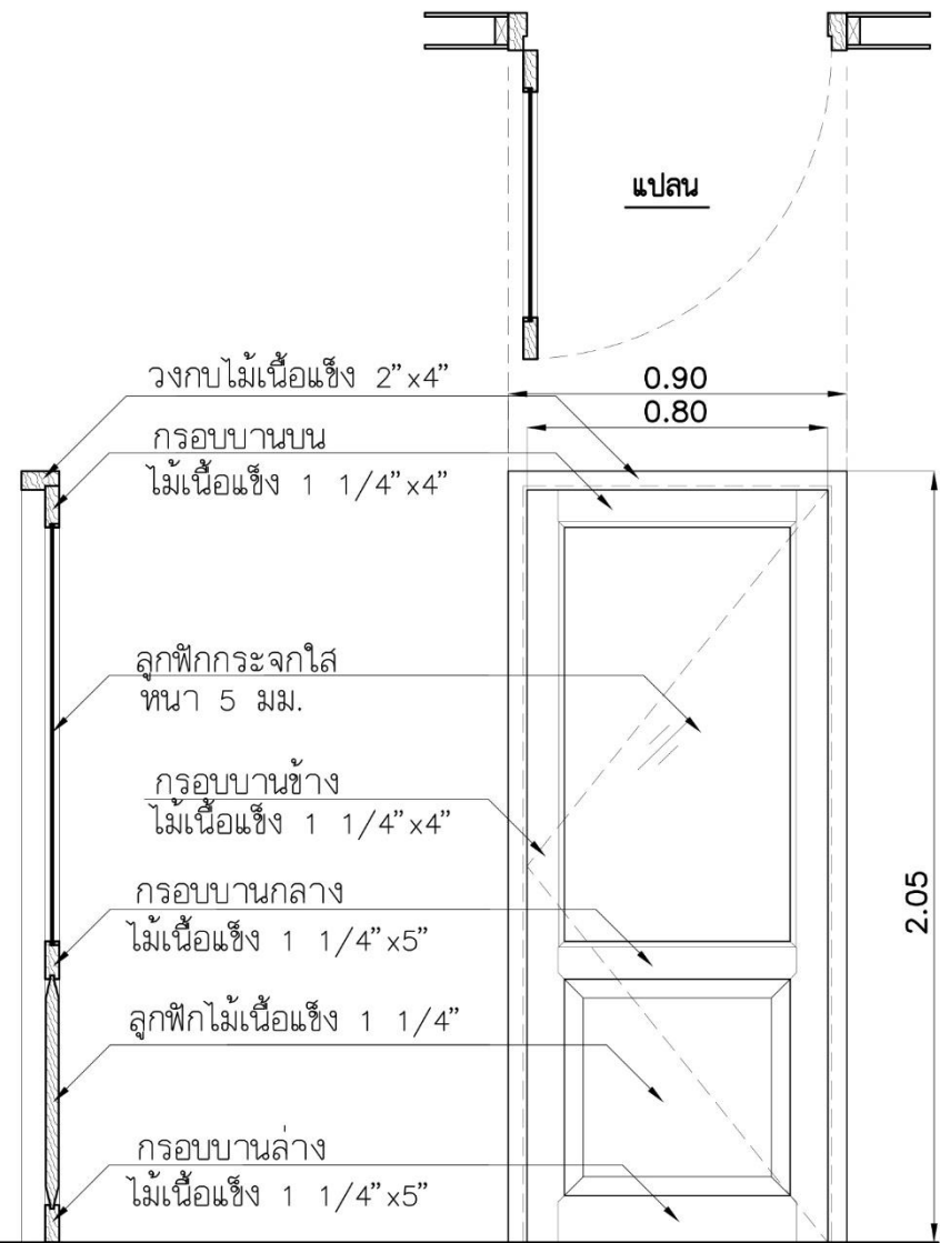
รูปตัด ประตูบานไม้เปิดเดี่ยว ชนิดบานลูกฟักกระจกและไม้
