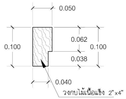
แบบขยายวงกบไม้ ใช้กับประตูทั่วไป
