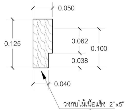
แบบขยายวงกบไม้ ใช้กับประตูห้องน้ำ
