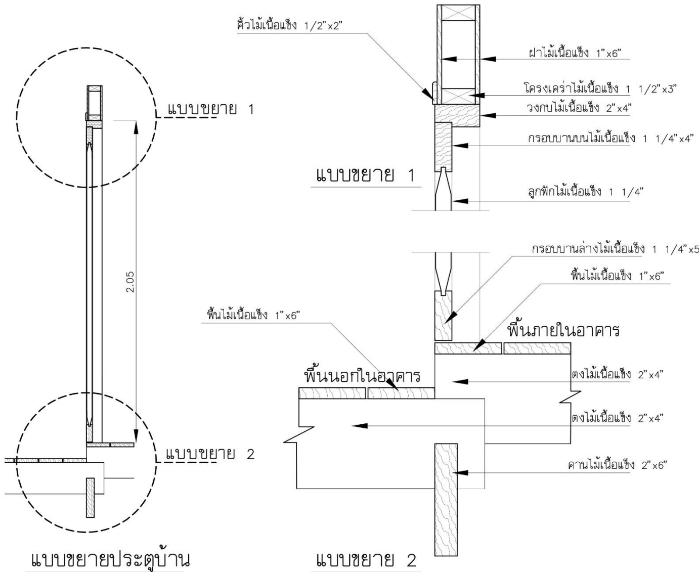
แบบขยายวงกบไม้ ใช้กับประตูทั่วไป
