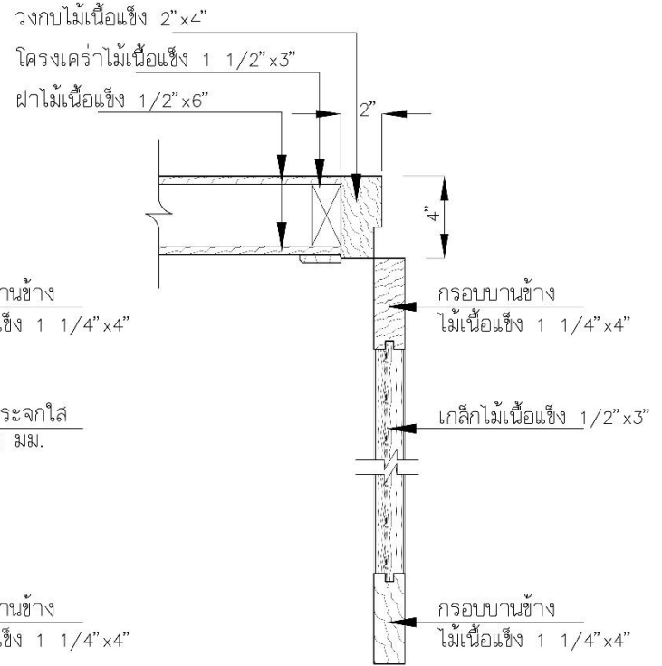
แบบขยายประตู ประตูบานเกล็ดไม้
