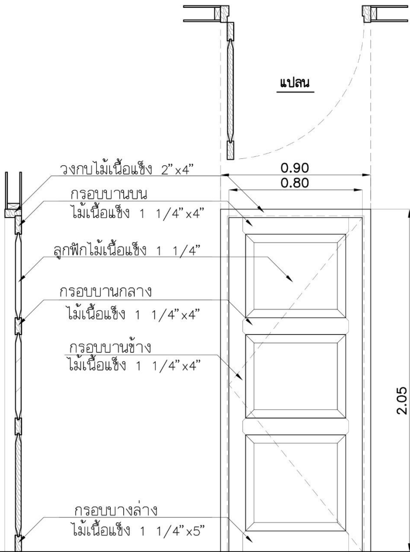
รูปตัด ประตูบานไม้เปิดเดี่ยว ชนิดบานลูกฟักไม้
