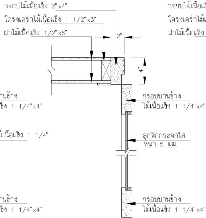
แบบขยายประตู ประตูบานลูกกระจก
