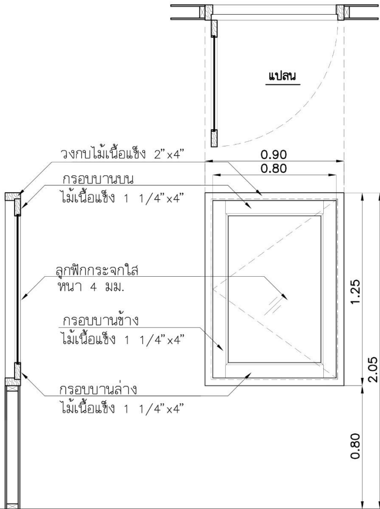
รูปตัด หน้าต่างบานไม้เปิดเดี่ยว น1 รูปด้าน ชนิดบานลูกพีกระจก
