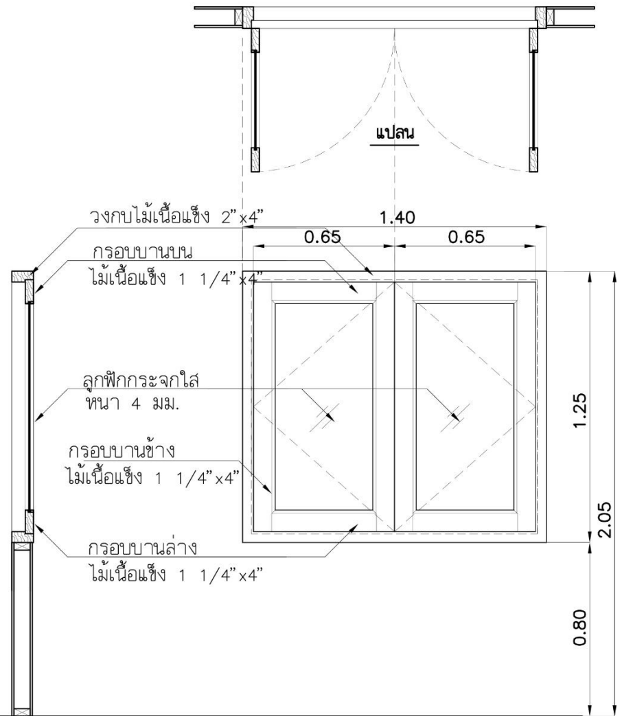
รูปตัด หน้าต่างบานไม้เปิดคู่ น2 รูปด้าน ชนิดบานลูกพีกระจก
