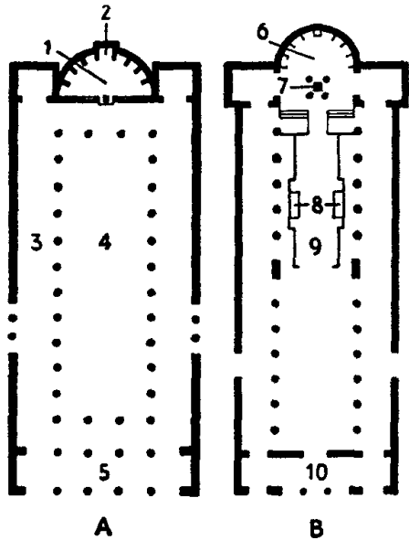
BASILICA: A. ROMAN BASILICA. B. EARLY CHRISTIAN BASILICA
