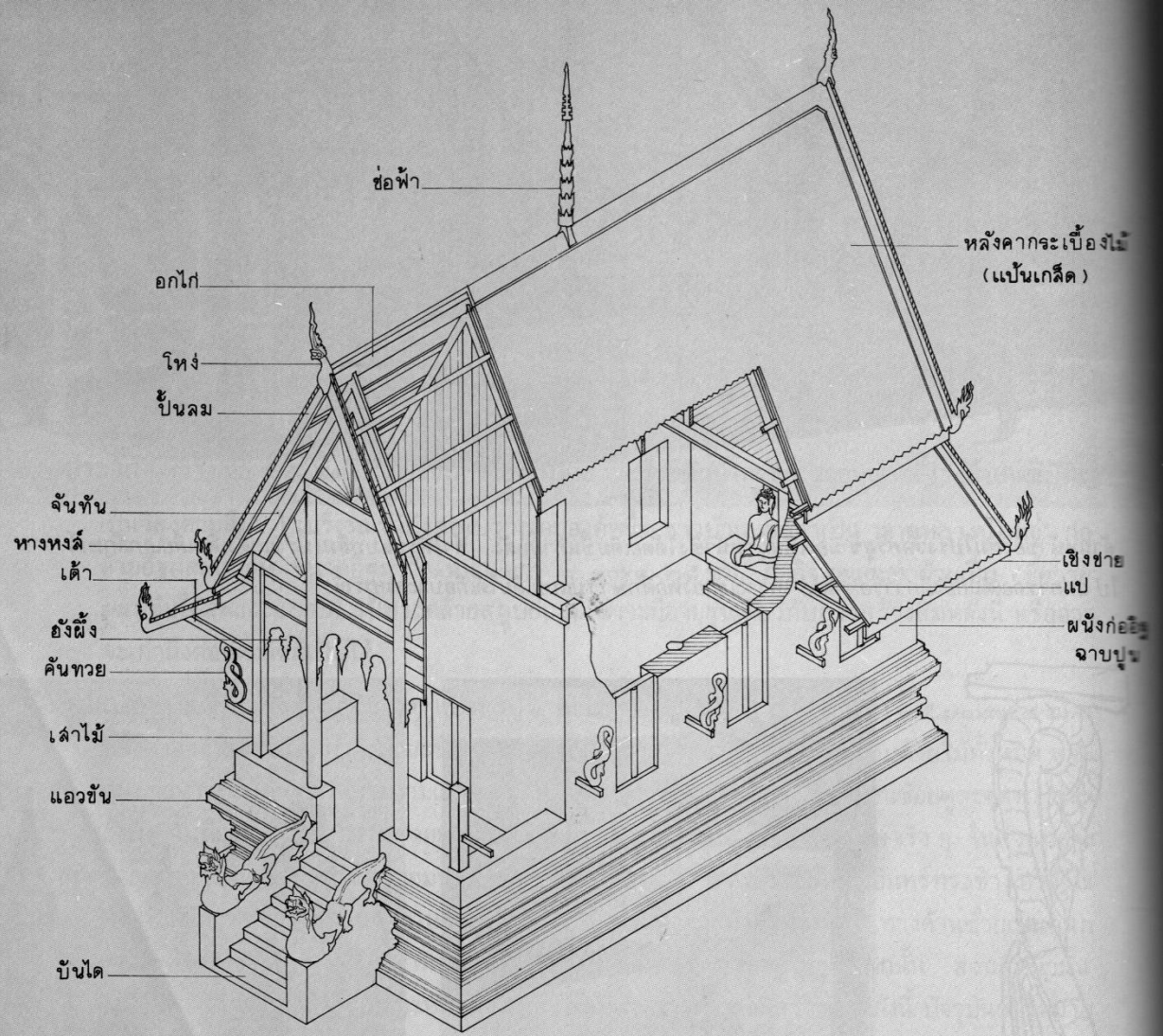
รูปตัดแสดงชั้นส่วนและชื่อเรียกของ “ลืออีสาน” (ชนิดลือทึบ)
