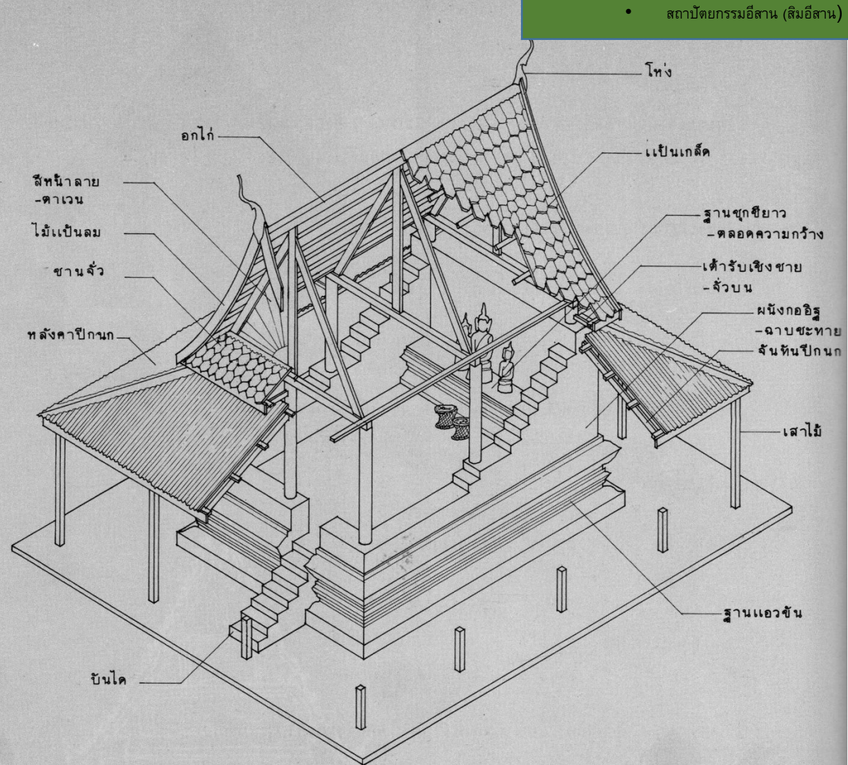
รูปตัดแสดงชั้นส่วนและชื่อเรียกของ “ลืออีสาน” (ชนิดลือโปร่ง)
