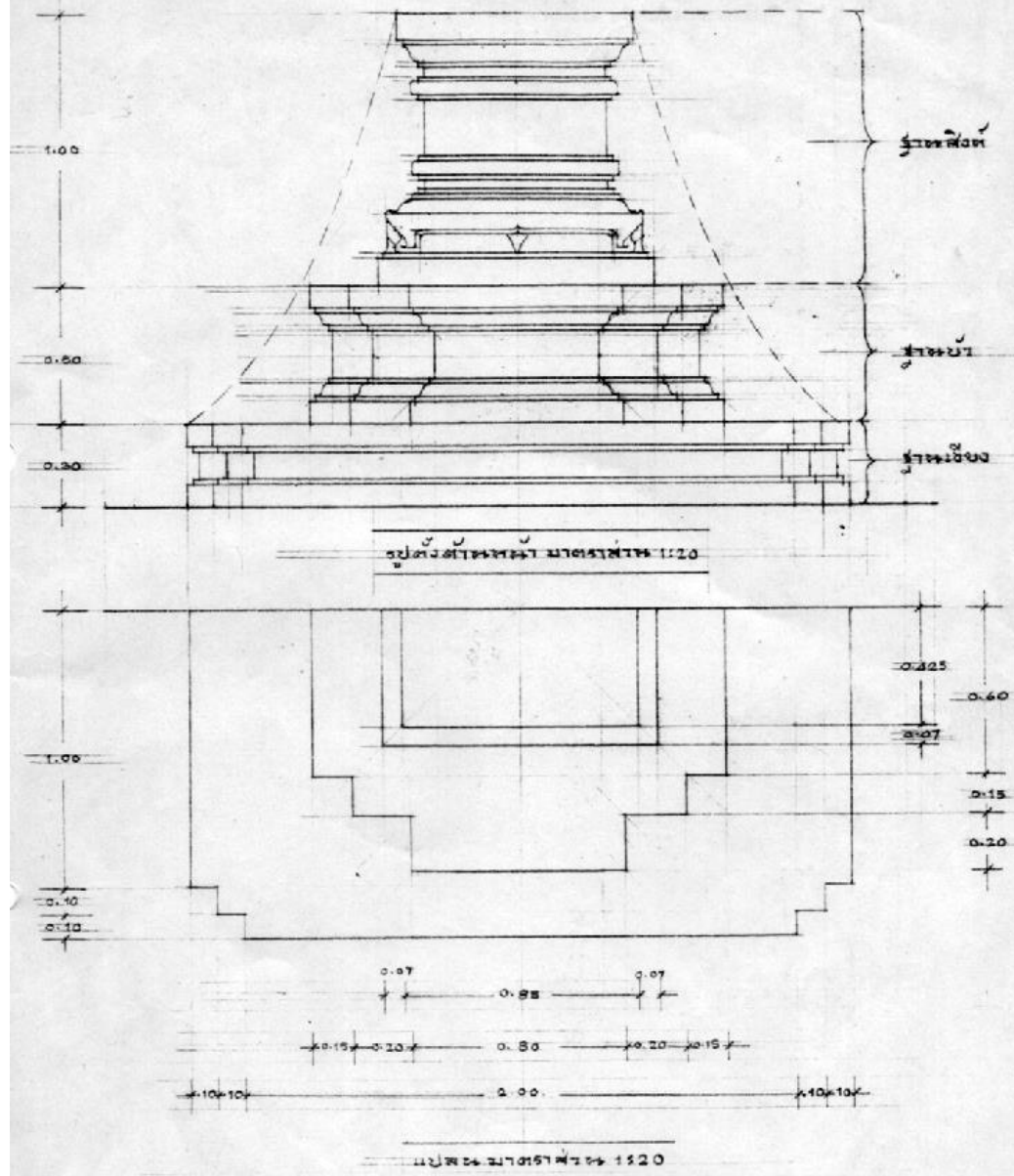
แบบแปลนสถาปัตย์ ฐานบัวกลมสี่เหลี่ยม เพื่อใช้รับองค์พระ หรือ รูปปั้น ซึ่งเกตุ รูปทรง และ การย่อขนาด
