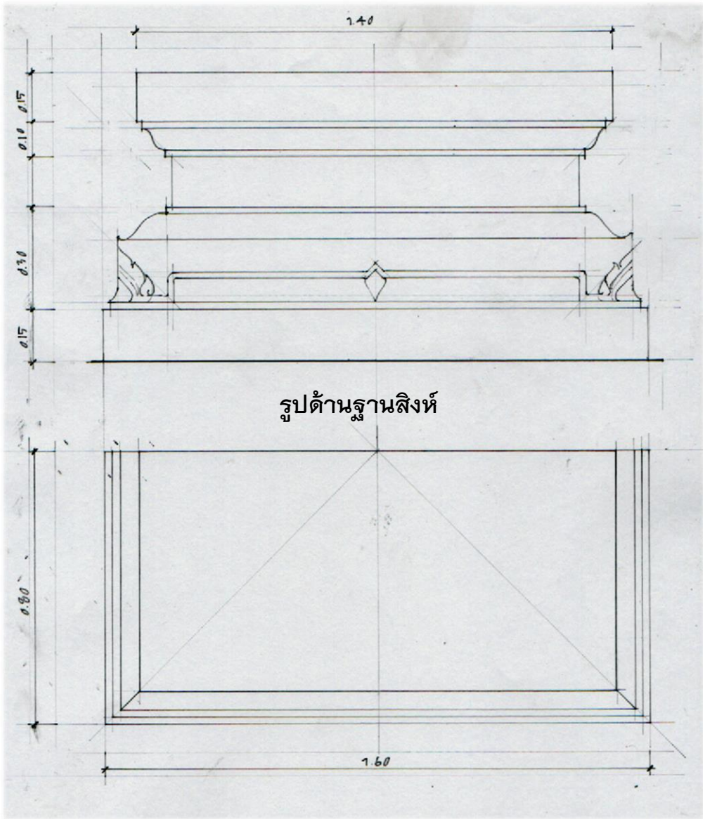
แปลนฐานสิงห์
