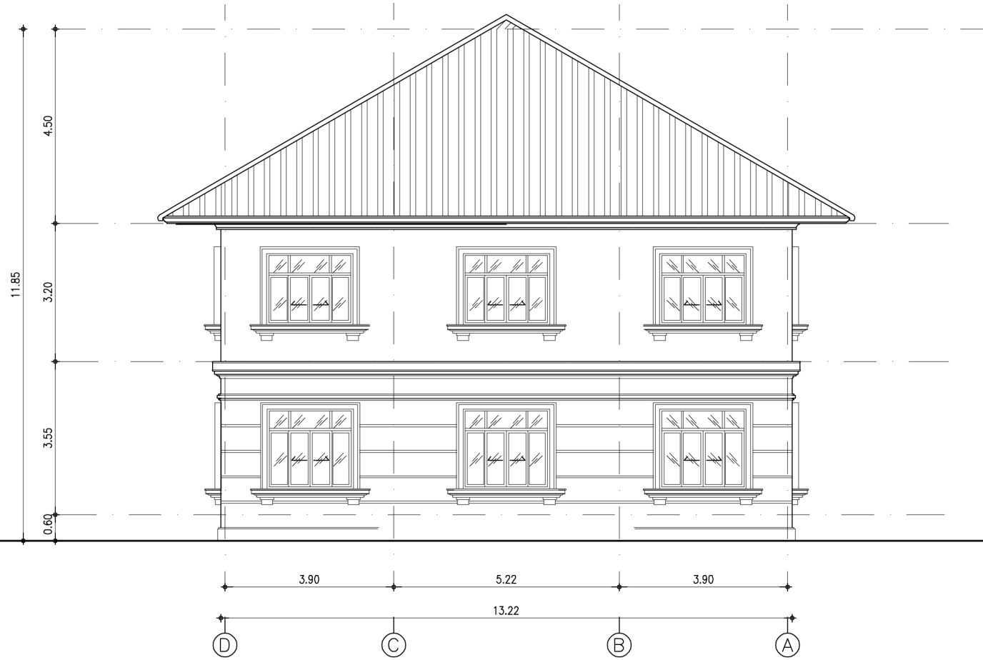
ELEVATION 3
