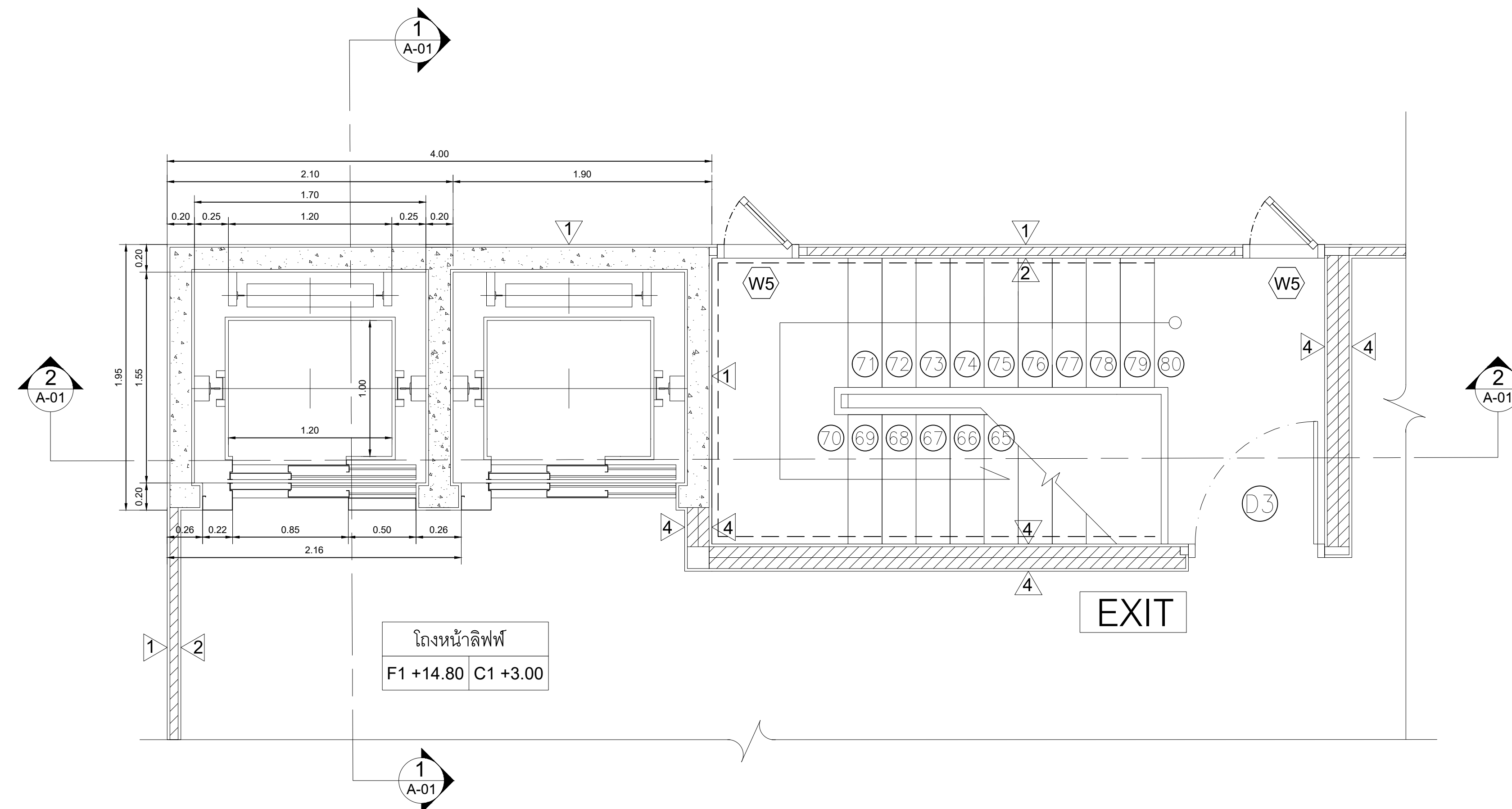
แบบขยายลิฟท์ ชั้น 5 Scale 1:25
