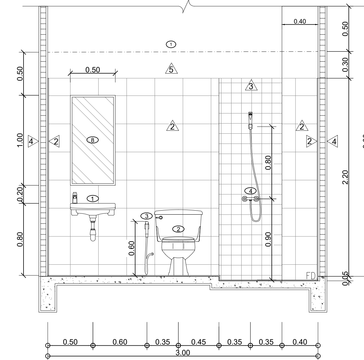
รูปตัด B Scale 1:25
