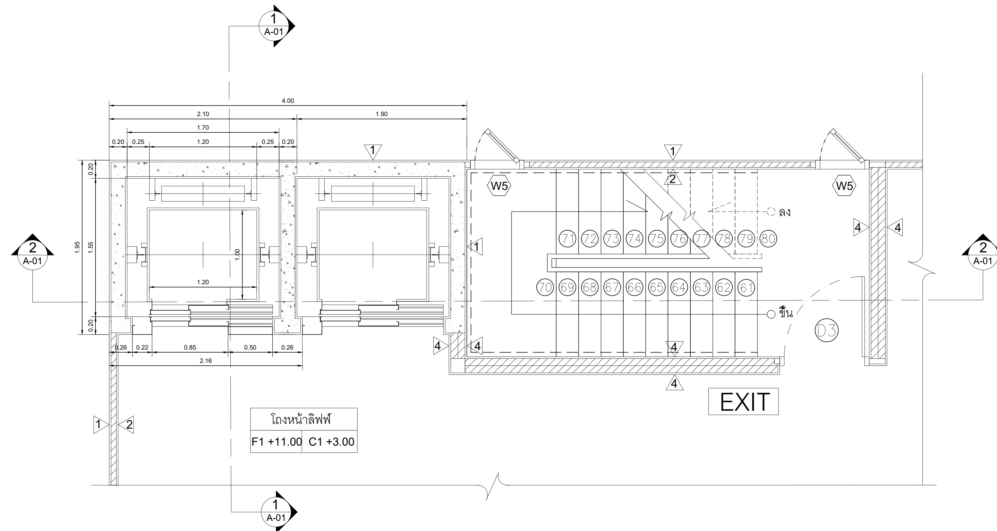
แบบขยายลิฟท์ ชั้น 4 Scale 1:25
