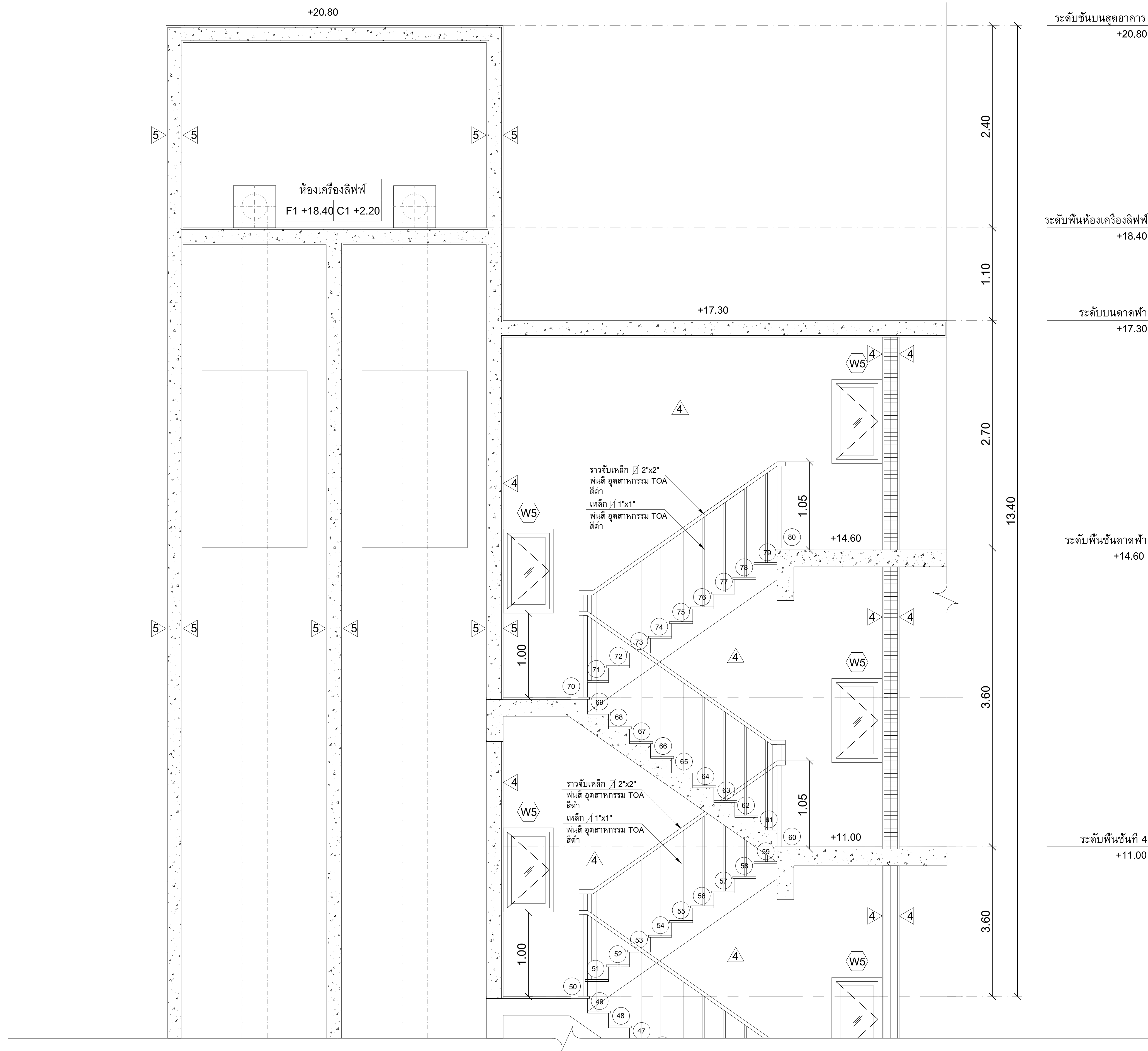
รูปตัดแบบขยายลิฟท์ ส่วนที่ 2 Scale 1:25
