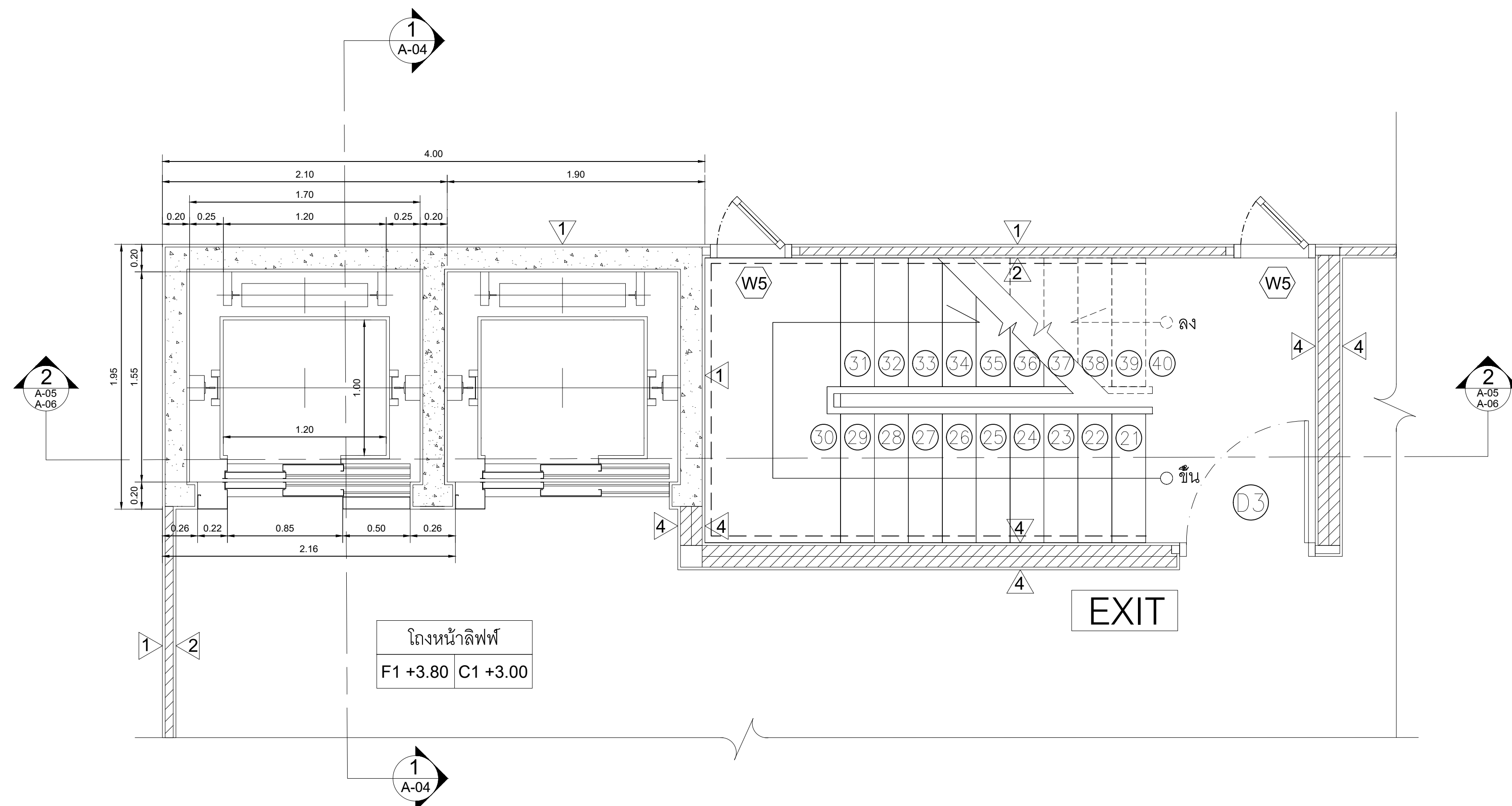
แบบขยายลิฟท์ ชั้น 2 Scale 1:25
