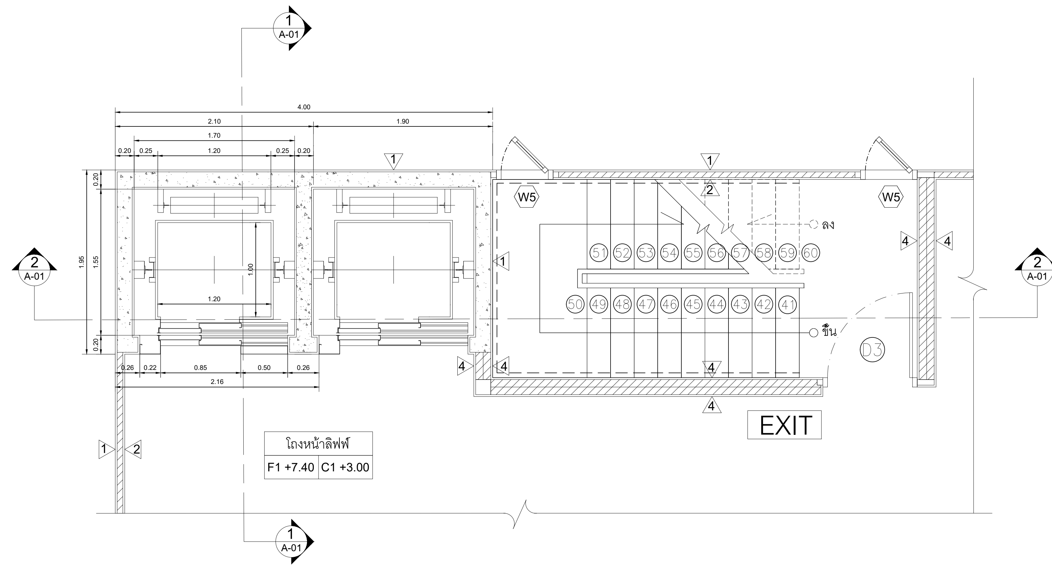
แบบขยายลิฟท์ ชั้น 3 Scale 1:25
