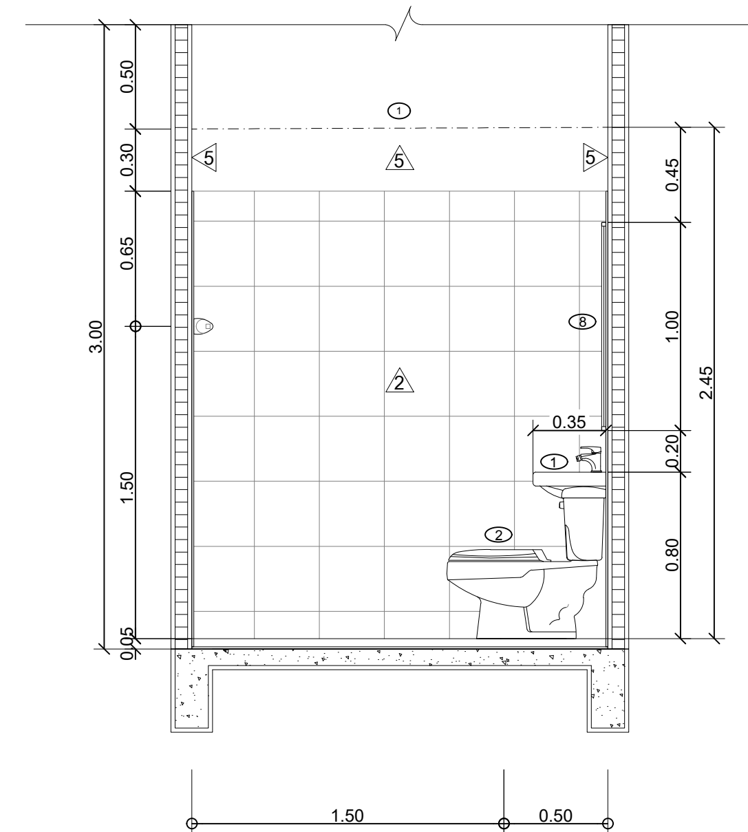
รูปตัด A Scale 1:25
