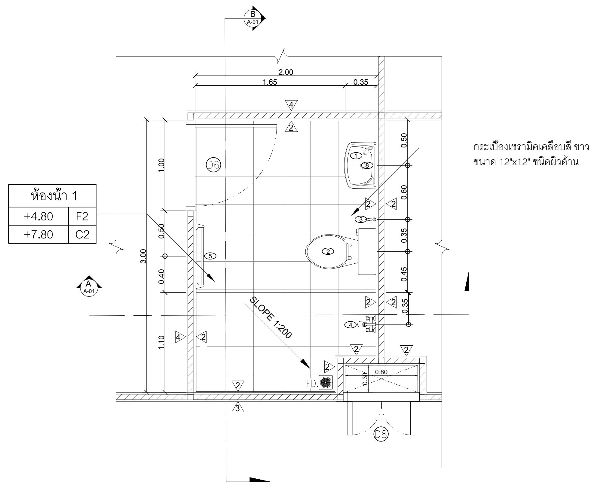
แบบขยายห้องน้ำ 1 Scale 1:25
