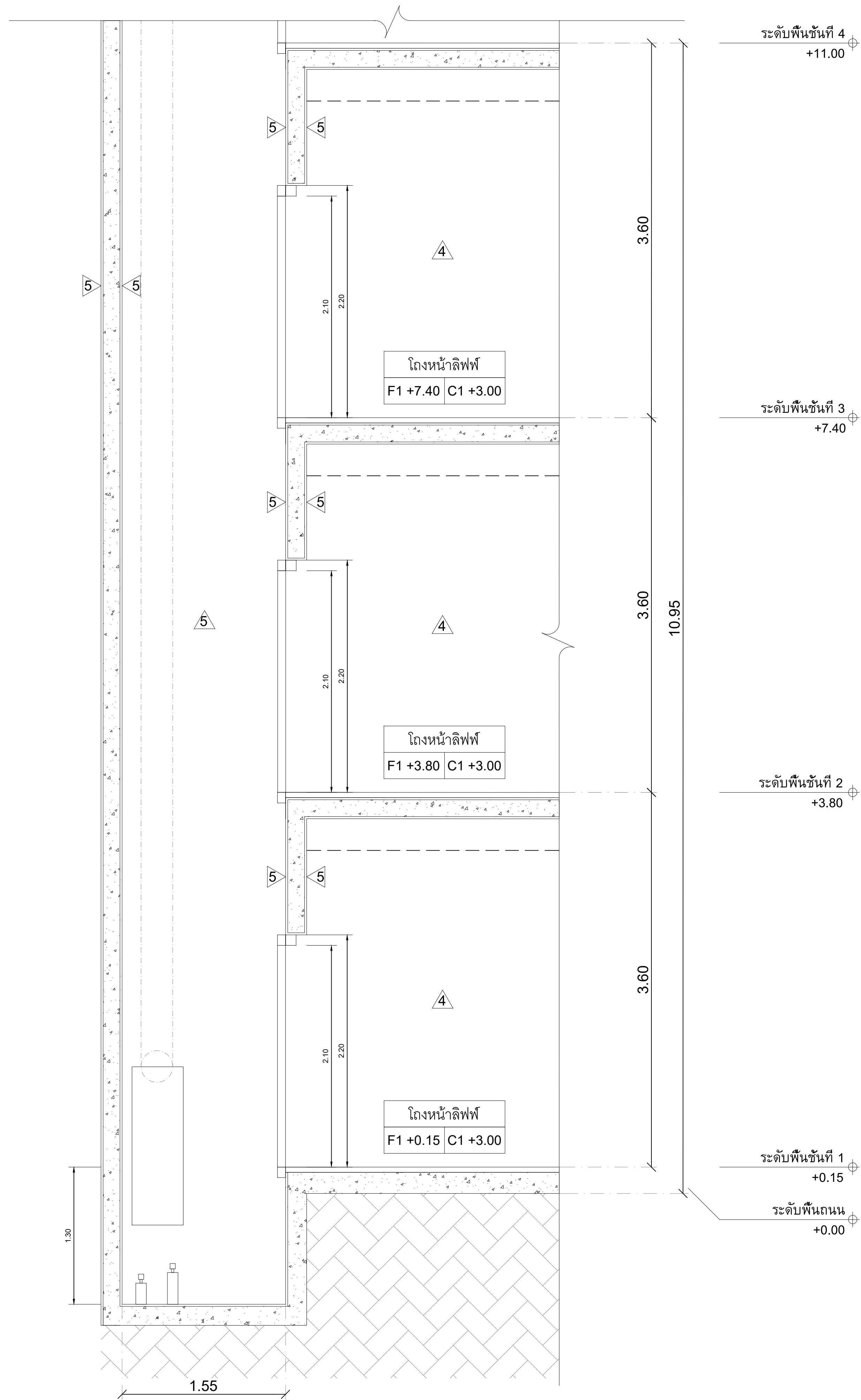
รูปตัดแบบขยายลิฟท์ ส่วนที่ 1 Scale 1:25
