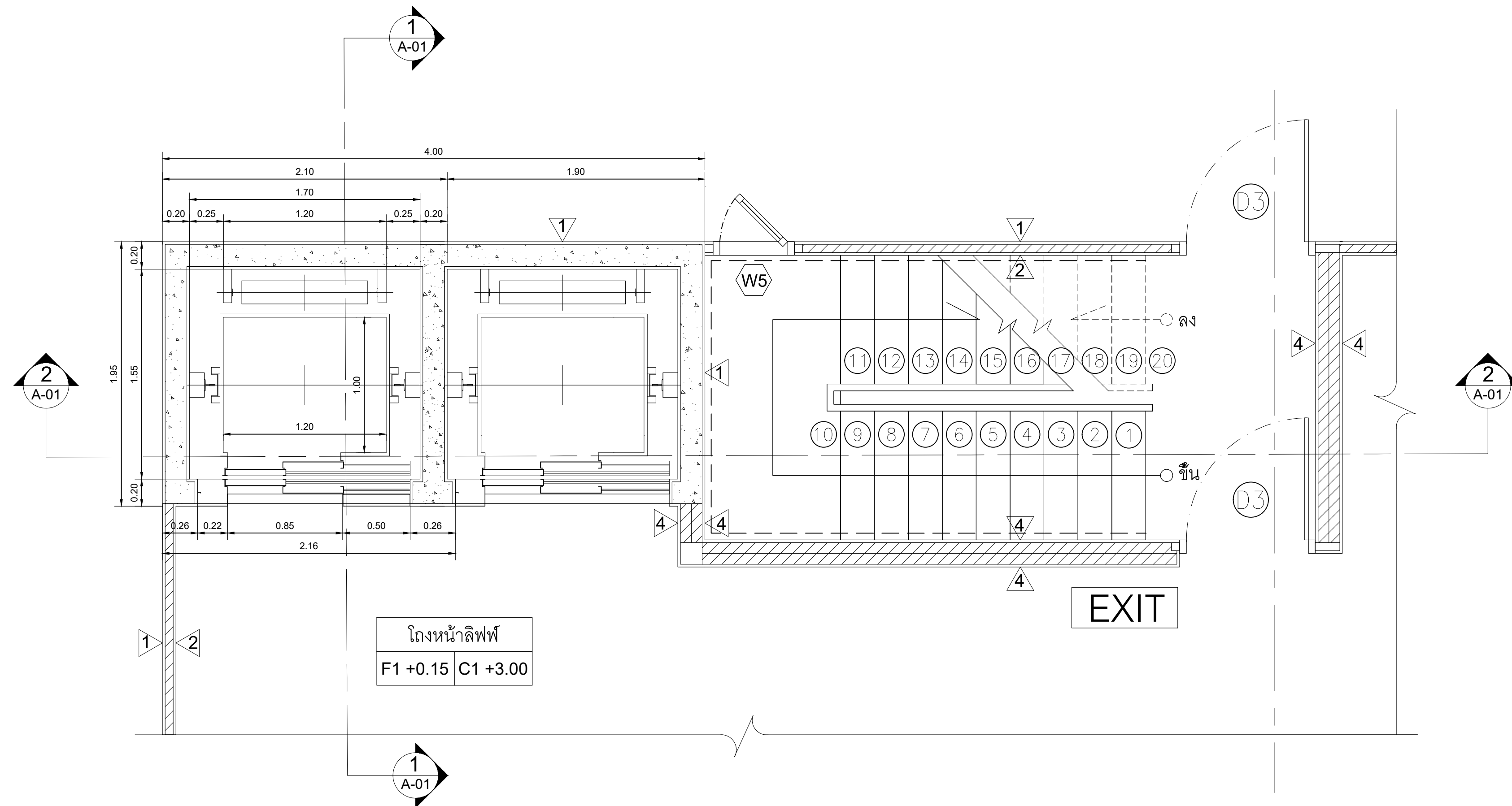
แบบขยายลิฟท์ ชั้น 1 Scale 1:25
