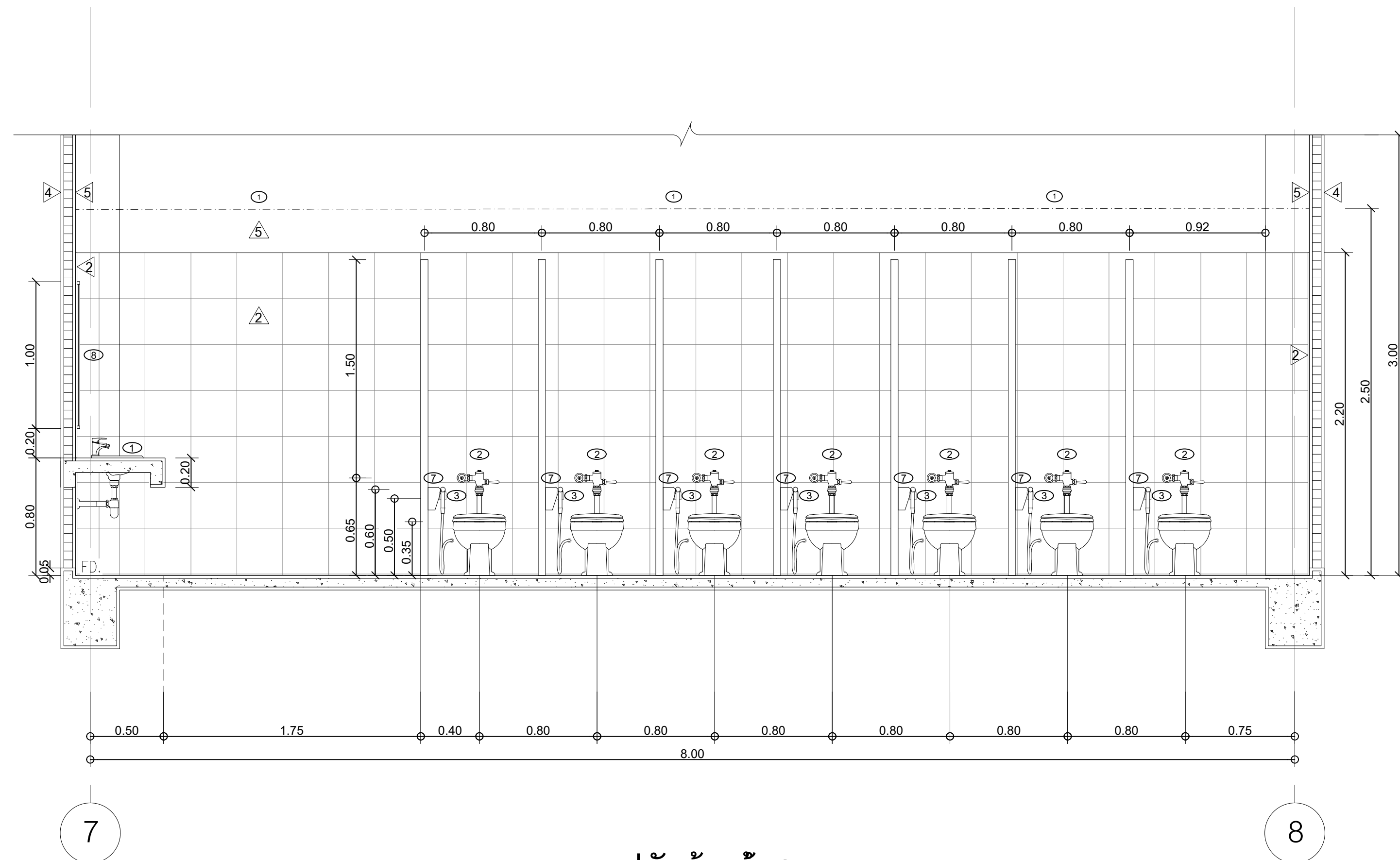
รูปตัดห้องน้ำ A Scale 1:25
